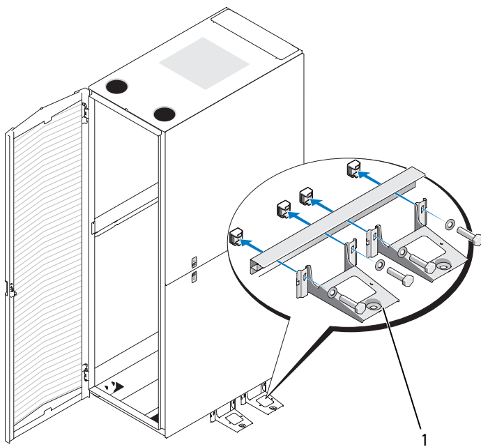
1 Seitliche Stabilisatoren (2)
